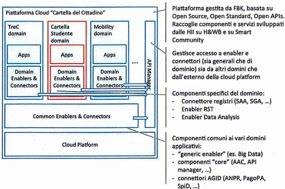
Figura 4 Architettura di riferimento
